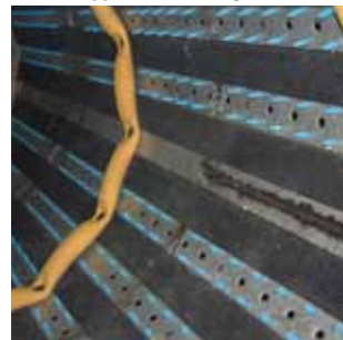
Kombination Bürste/Noppenauskleidung
